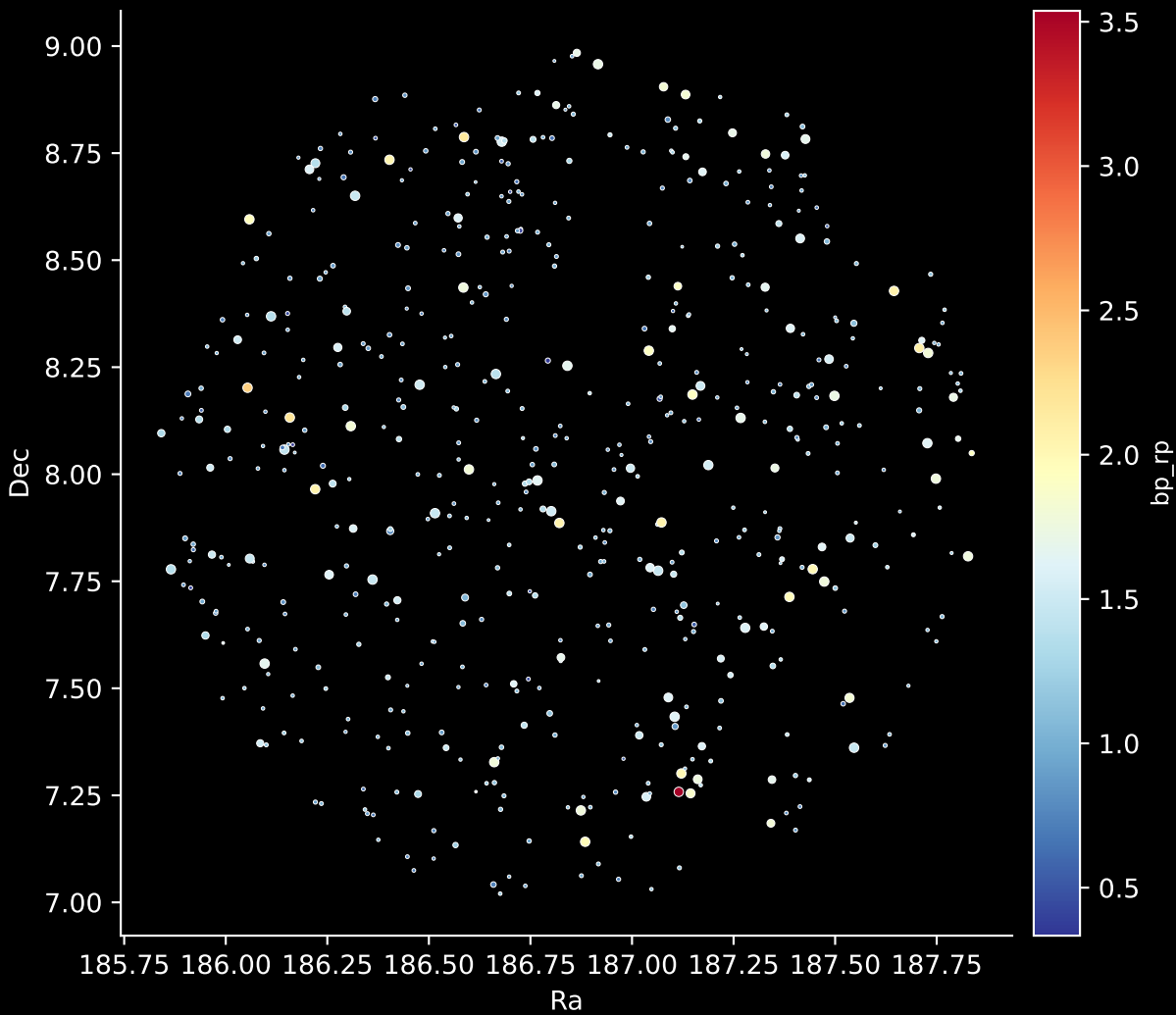
GALAH DR4 Field: [9466] Stars: 546
