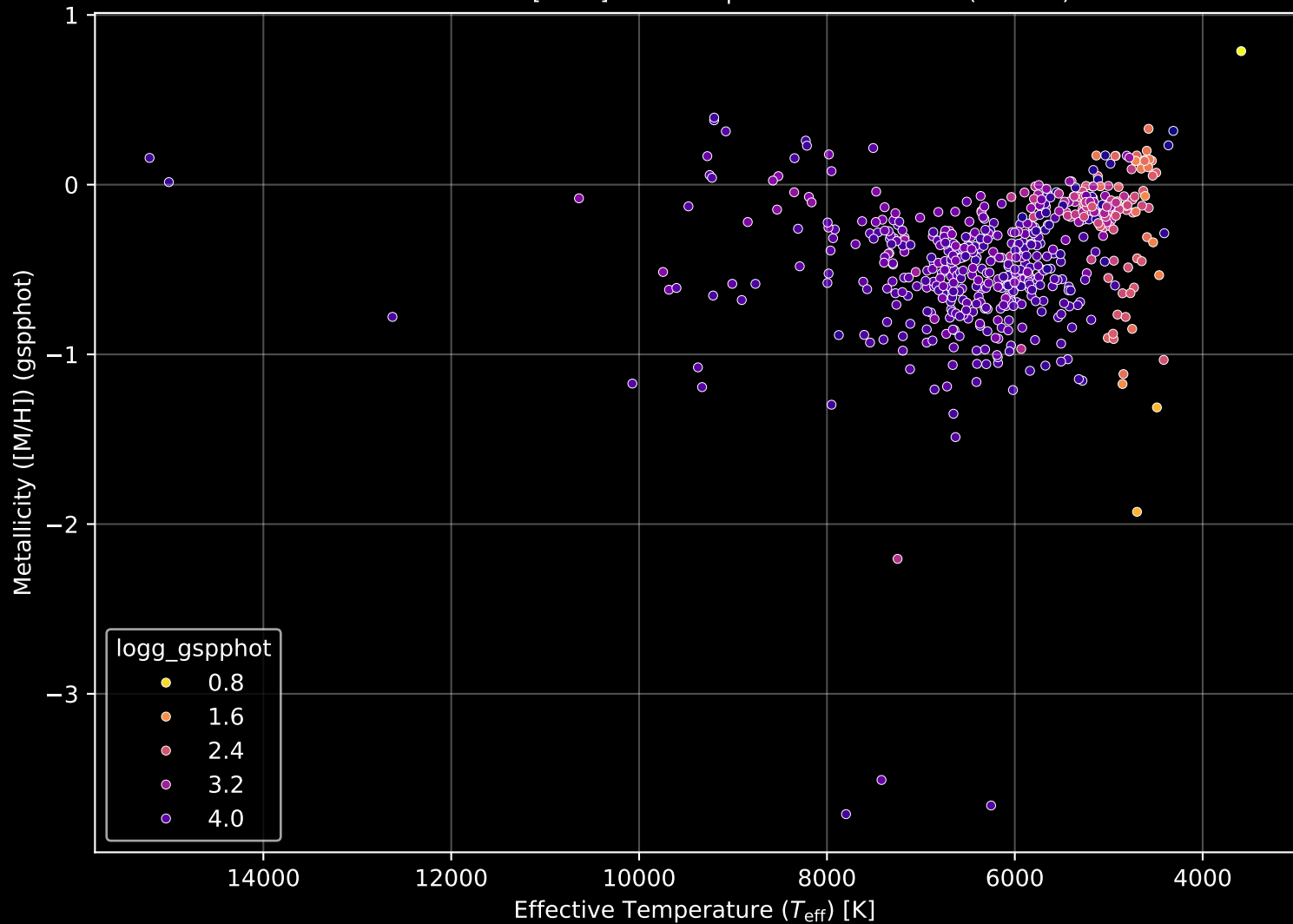
GALAH DR4 Field: [9466] Stellar Population Parameters (n= 546)
