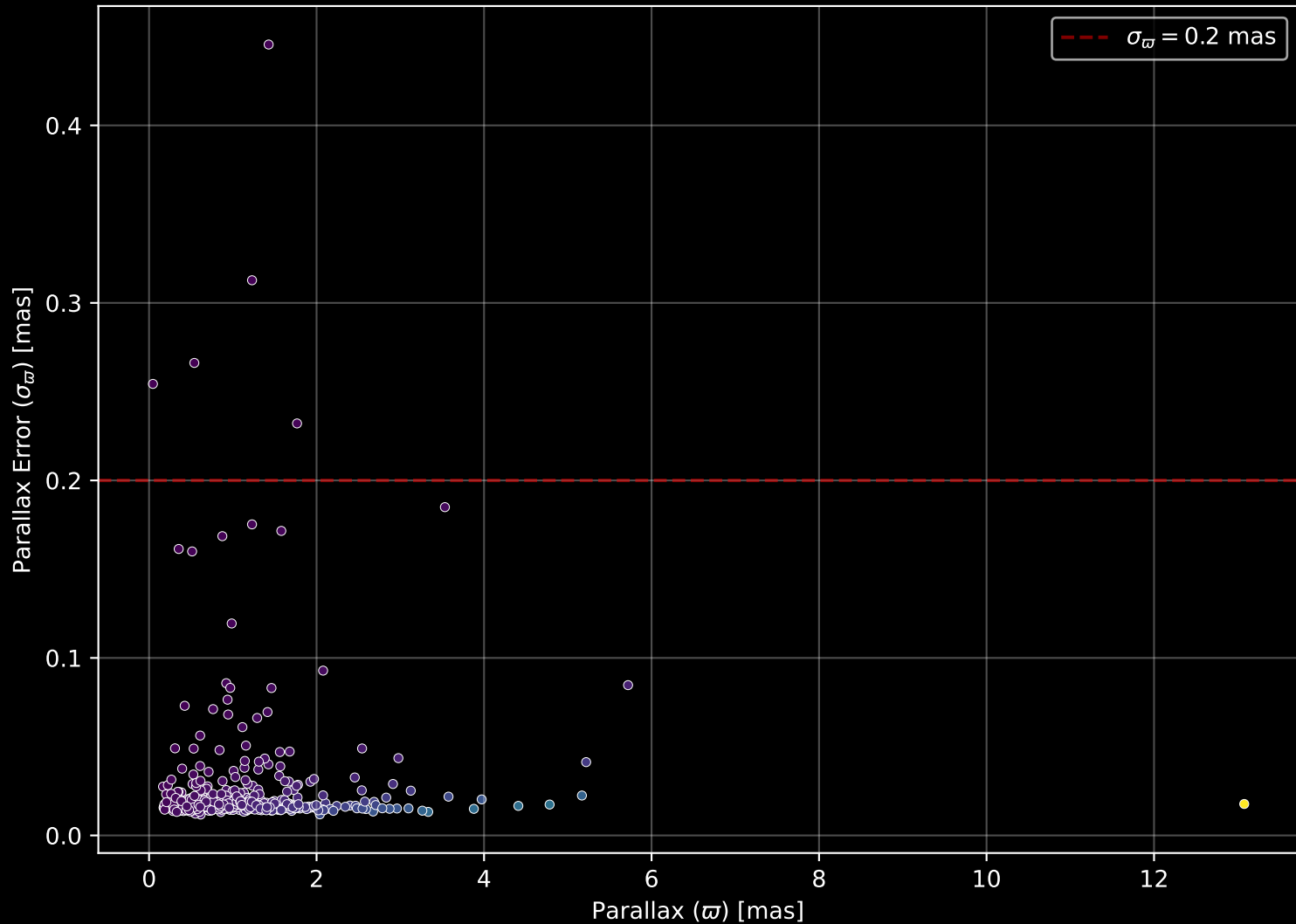
GALAH DR4 Field: [9466] Parallax Quality (n= 546)
