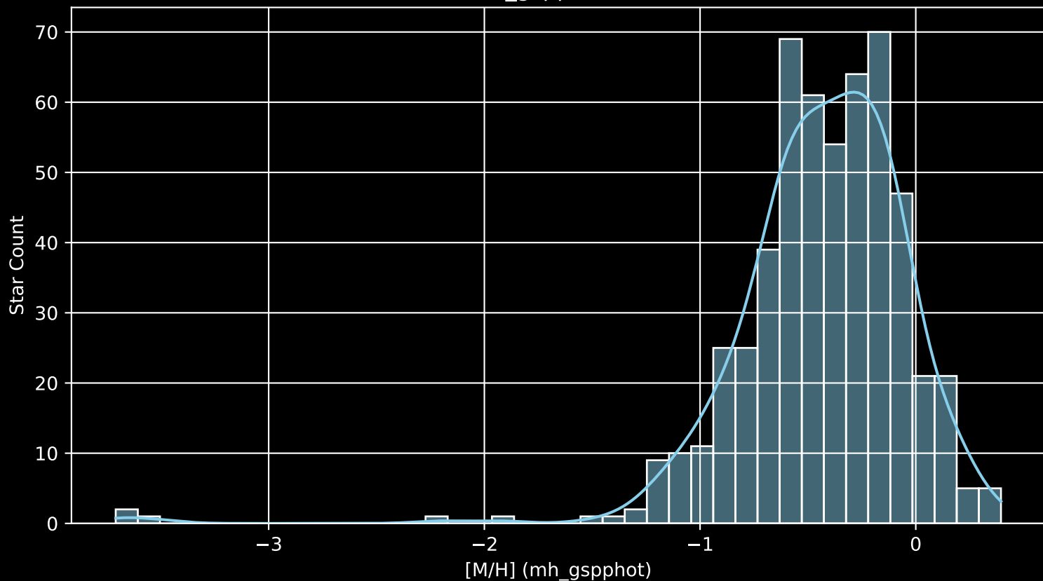
GALAH DR4 Field: [9466] [M/H] (mh_gspphot) (n= 545)
